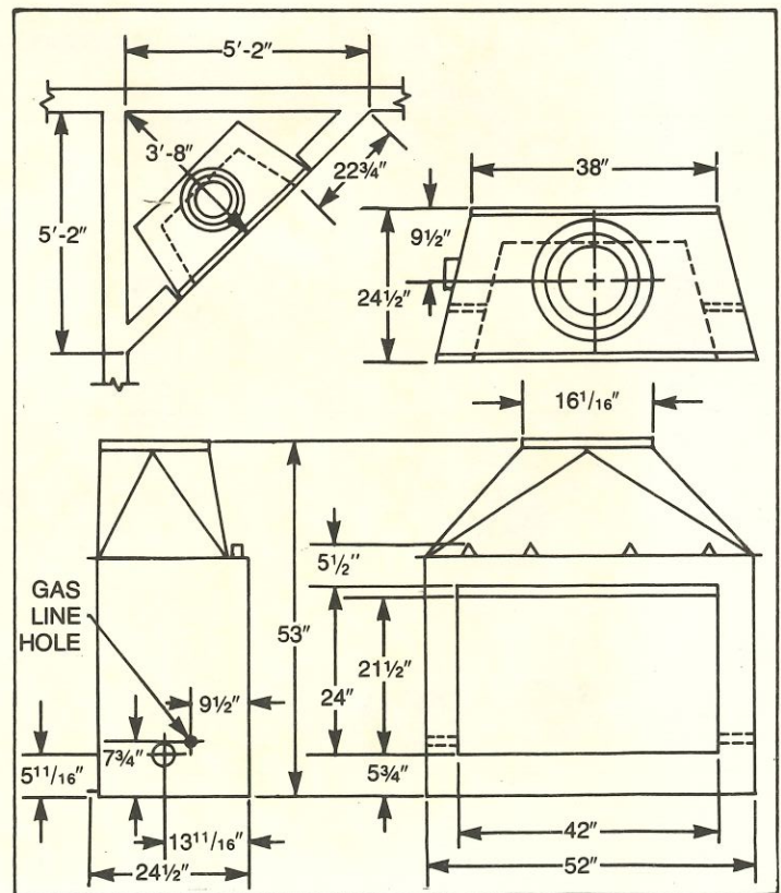
Fig. 26. Dimensions of MD42-AO.
