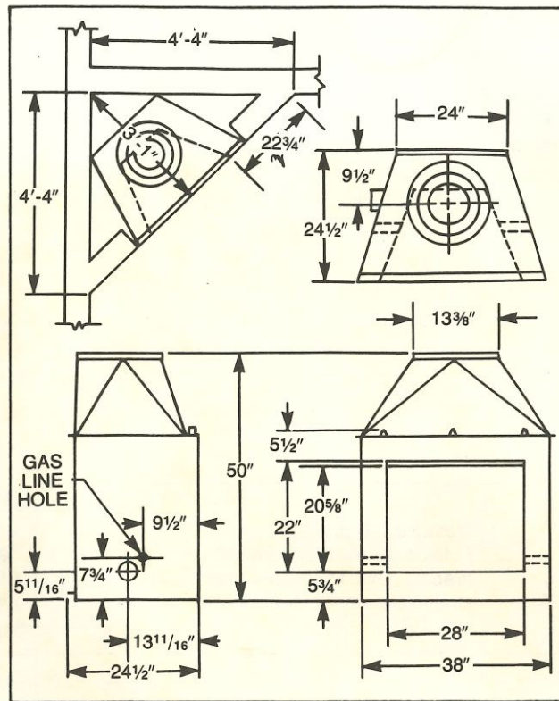
Fig. 24. Dimensions of M28-AO.
